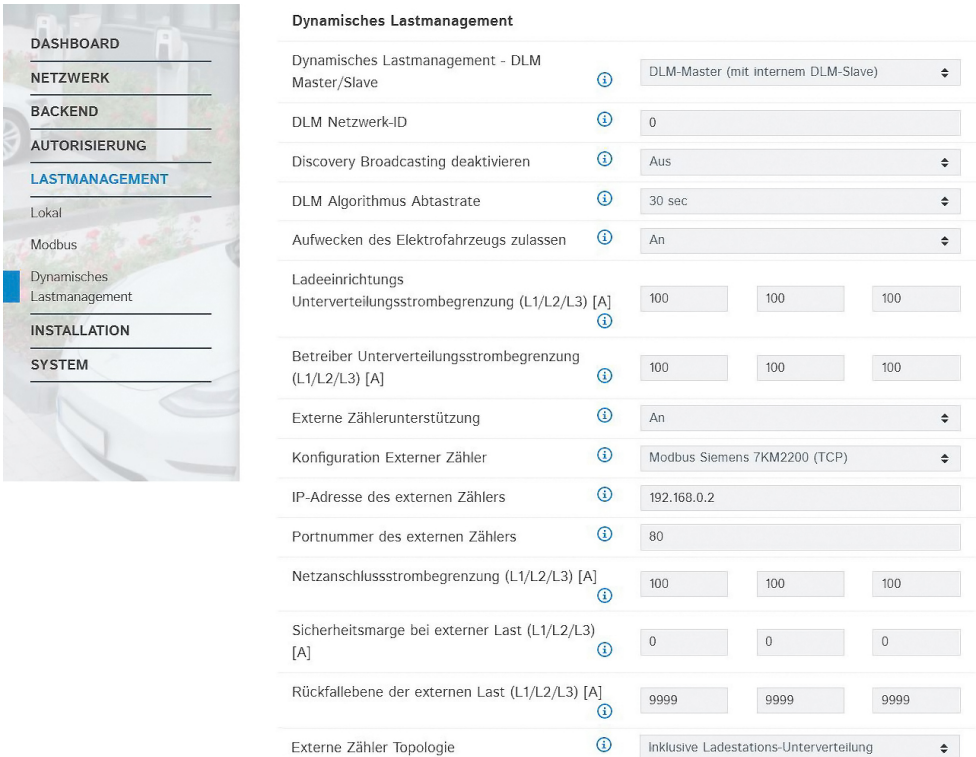
Abb. 22: Weboberfläche des DLM-Masters zur Konfiguration von Lastmanagement
