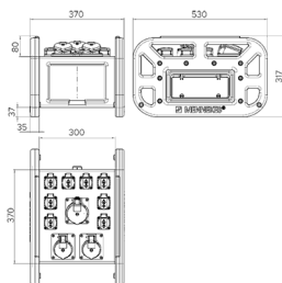
Zeichnung 5 MB 72 Maße in mm
