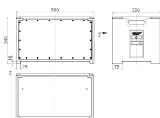
Zeichnung 5 MB 70 Maße in mm
