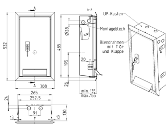
Zeichnung 5 MB 50 Maße in mm
