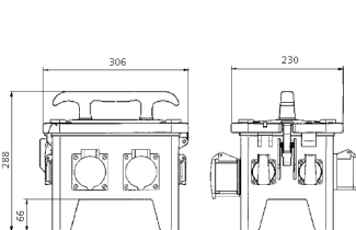
Zeichnung 5 MB 48a Maße in mm
