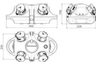
Zeichnung 1 MB 441 Maße in mm
