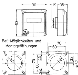
Zeichnung 1 MB 305 Maße in mm
