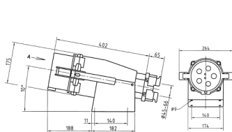
Zeichnung 2 MB 200/1 Maße in mm
