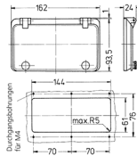
BestellNr. 40978 / Zeichn. 6 MB 15 / 8 TE
