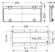
BestellNr. 40980 / Zeichn. 6 MB 14 / 12 TE
