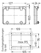
BestellNr. 40985 / Zeichn. 6 MB 16 / 6 TE
