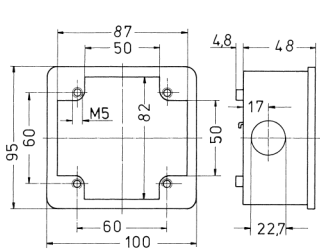
Zeichnung 1 MB 232 Maße in mm
