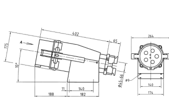
Zeichnung 2 MB 200/1
