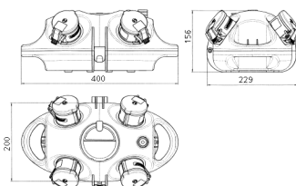
Zeichnung 1 MB 441 Maße in mm
